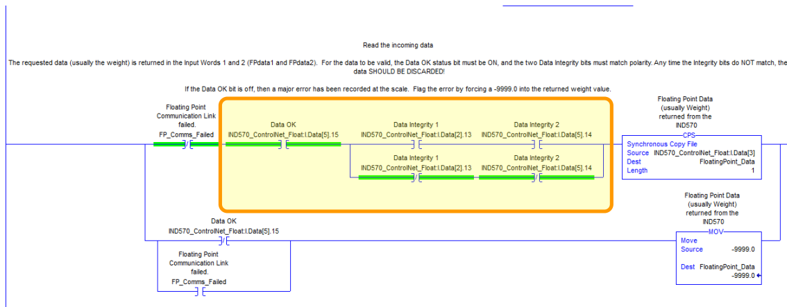
Abbildung 5-2: Korrekter Filterkontaktplan für Gleitpunktdaten
