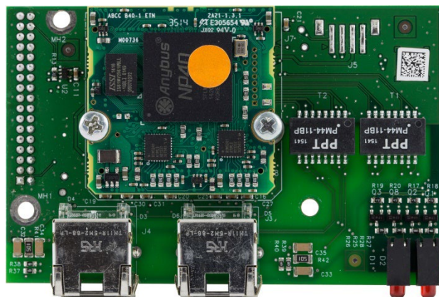
Abbildung 7-1: PROFINET-Modul
