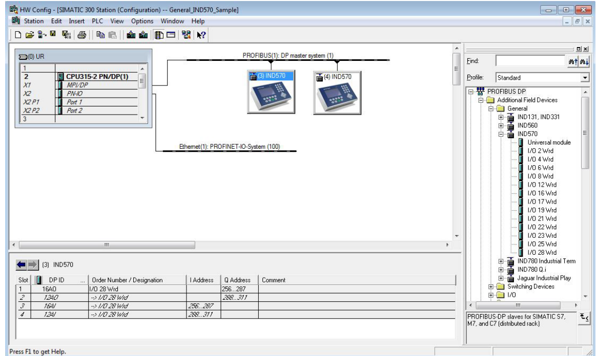
Abbildung 6-9: Hardware-Konfiguration
