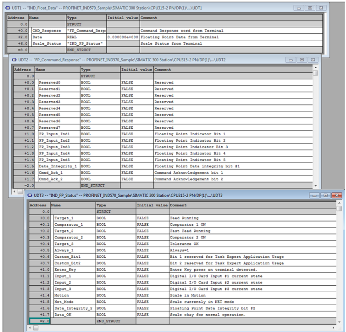
Abbildung 7-19: Im Gleitpunkt-Beispielprogramm verwendete UDT-Definitionen
