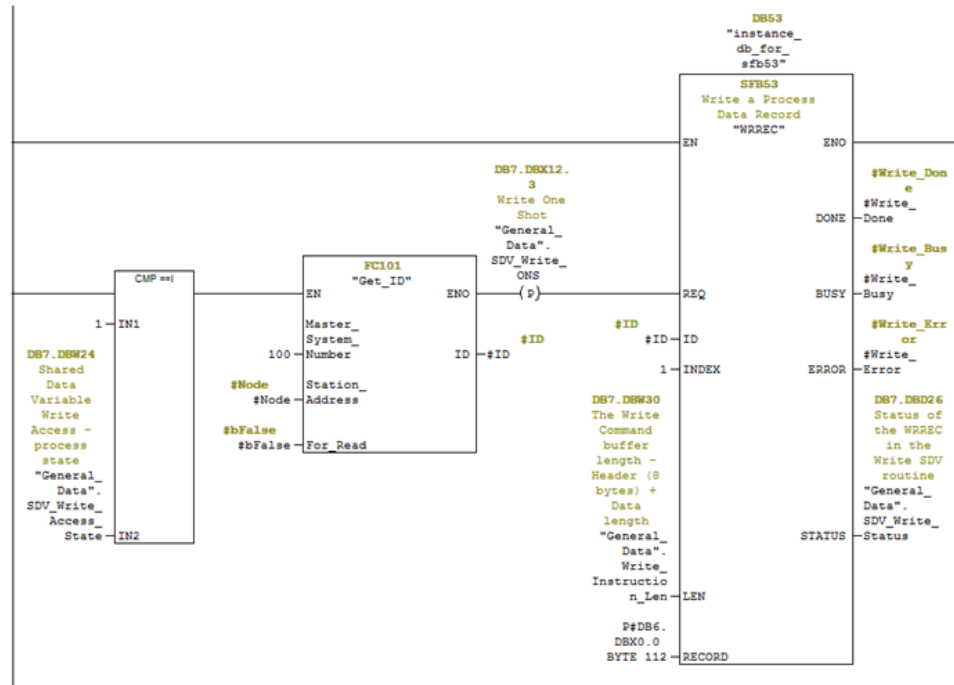
Abbildung 7-49: Netzwerk 2 von FB4
