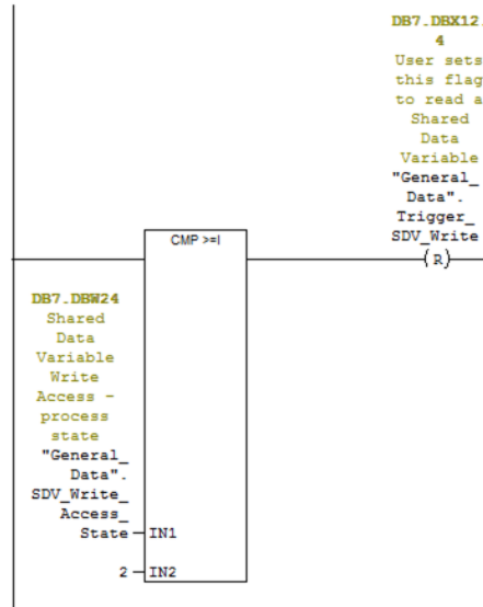
Abbildung 7-51: Netzwerk 4 von FB4
