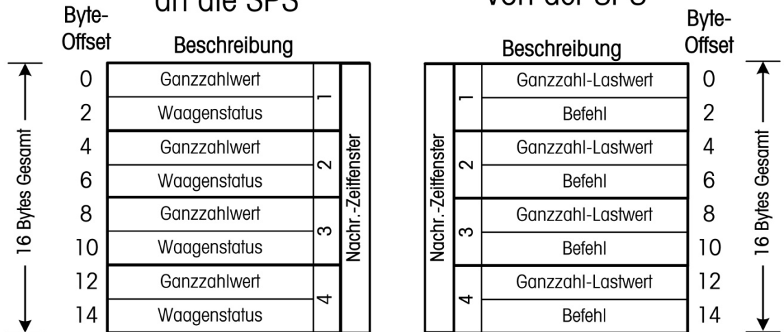
Abbildung 7-7: I/O-Zuordnung für Nachrichtenzeitfenster im Format Ganzzahl/Teilstrich
