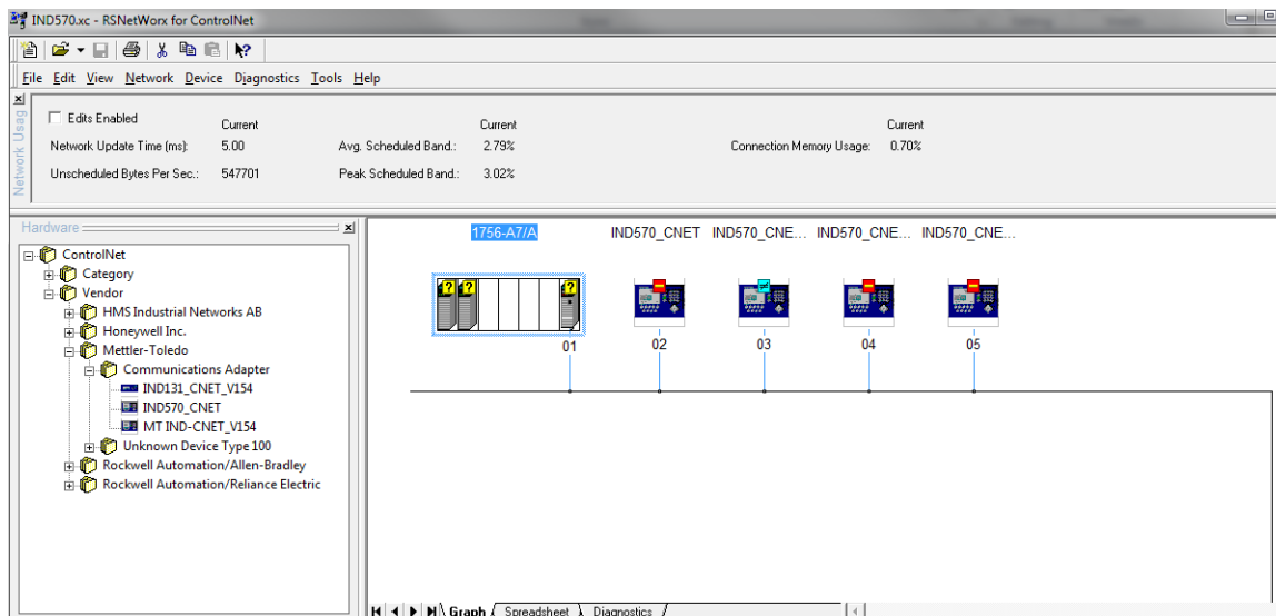
Abbildung 2-9: RSNetworx-Konfigurationsdatei mit 4 definierten Knoten
