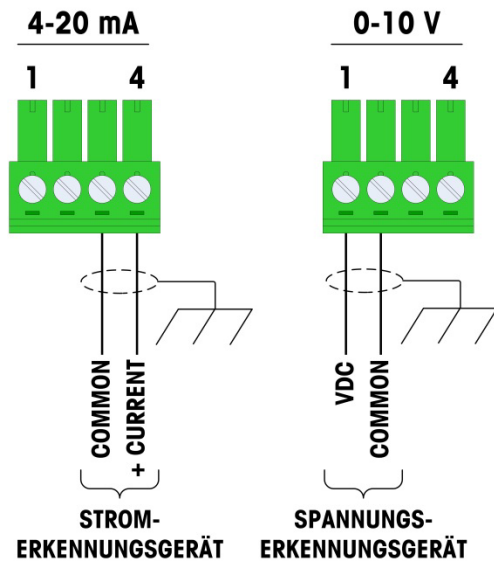
Abbildung 1-3: Verdrahtungsanschlüsse der Analogausgangs-Optionsplatine
