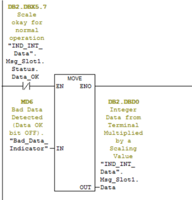
Abbildung 7-36: Netzwerk 4 von FC2
