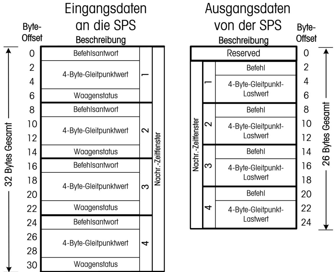
Abbildung 7-8: I/O-Zuordnung für Nachrichtenzeiträume im Format Gleitpunkt
