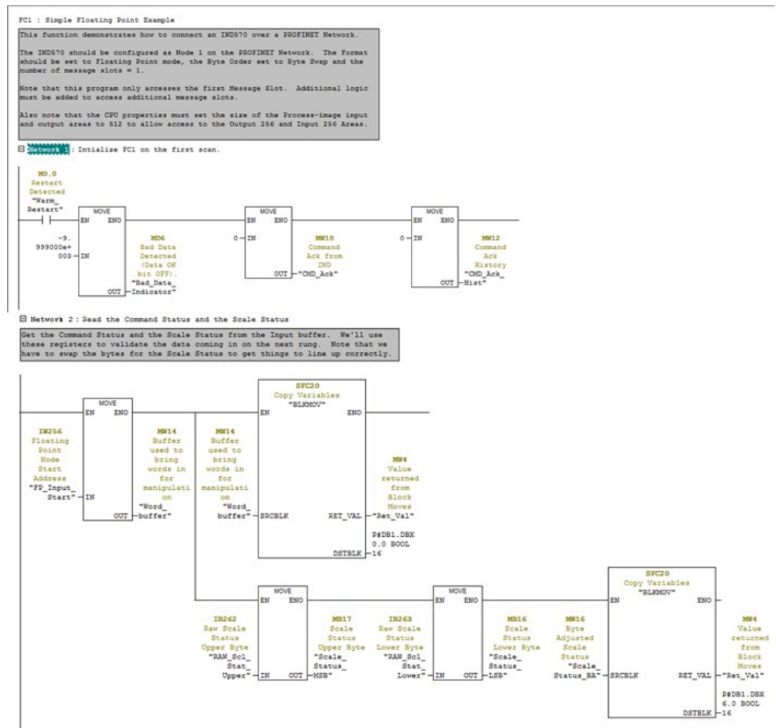
Abbildung 7-21: Netzwerke 1 & 2 von FC1
