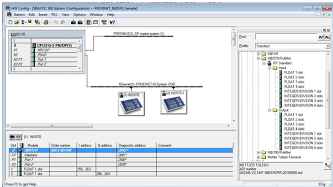
Abbildung 7-10: Hardware-Netzwerksetup (aktive Referenz erforderlich)
