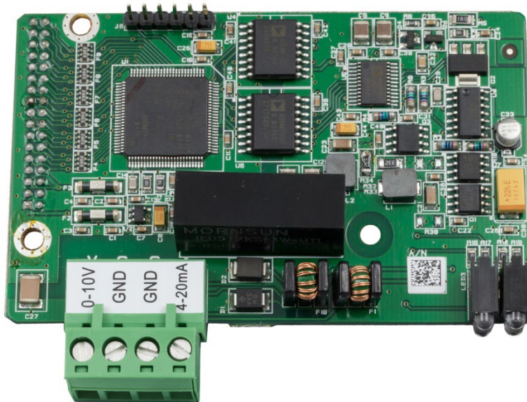
Abbildung 1-1: Analog-Ausgangs-Optionsplatine
