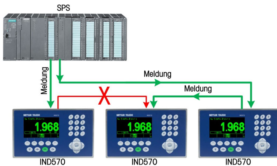
Abbildung 7-6: Unterbrochener MRP-Ring
