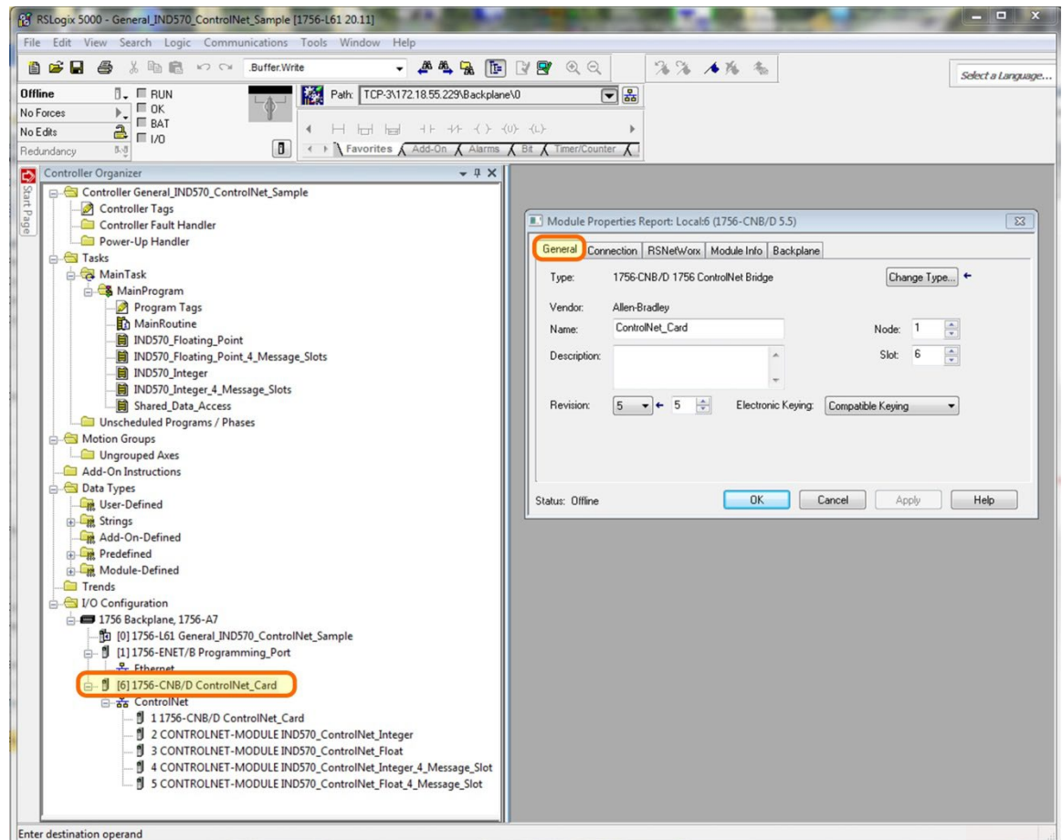
Abbildung 2-6: 1756 CNB-Konfiguration
