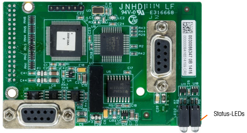
Abbildung 6-1: PROFIBUS-Optionsplatte für aggressive Umgebungen
