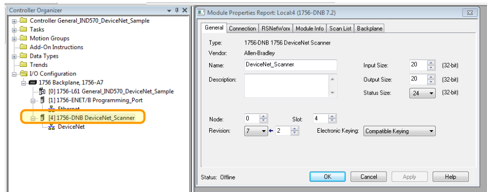
Abbildung 3-23: DeviceNet-Scannermodul-Konfiguration
