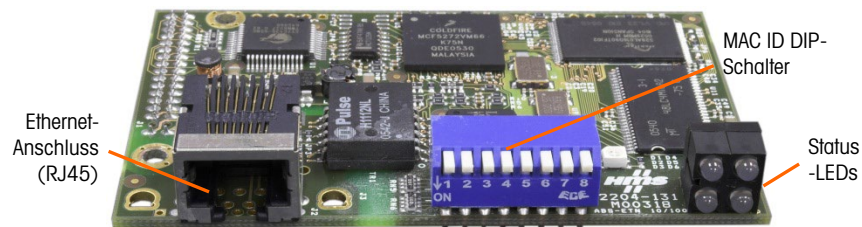
Abbildung 4-1: Ethernet/IP-Modulkomponenten
