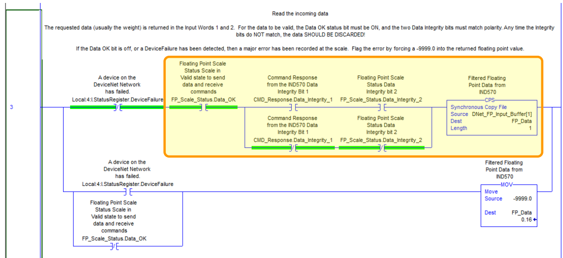
Abbildung 3-26: Filtern der Gleitpunktdaten in die PLC
